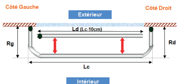
Rail KSC - 2 angles 90° : 1 ou 2 rideaux + voilage
