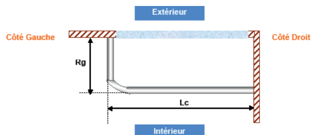
Rail KSC - 1 angle à 90° (Retour Gauche) : 1 Rideau
