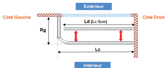
Rail KSC - 1 angle à 90° (Retour Gauche) : 1 Rideau + voilage
