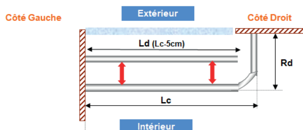
Rail KSC - 1 angle à 90° (Retour droit) : 1 Rideau + voilage
