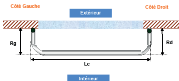
Rail KSC - 2 angles 90° : 1 ou 2 rideaux
