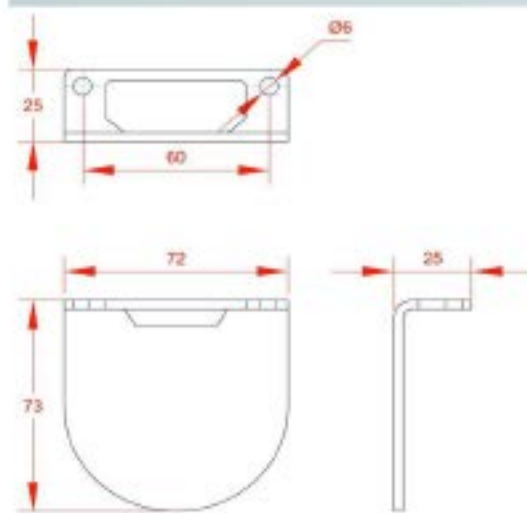
Equerre 73 x 72
