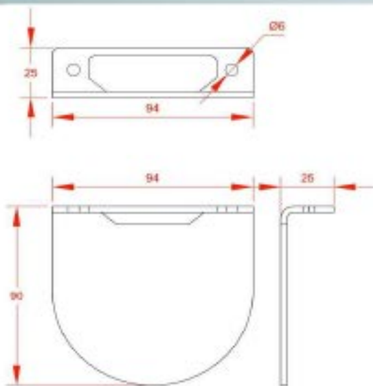
Equerre 90 x 94
